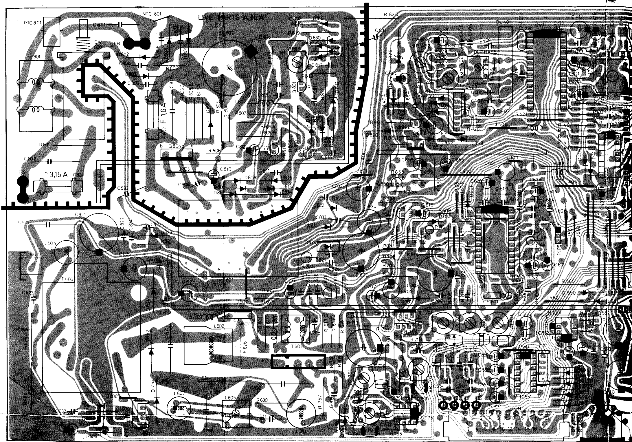
SIGNAL P.C.B.
